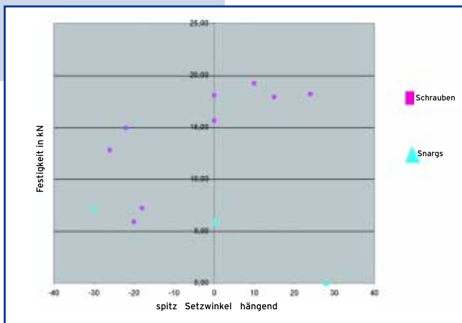
Diagramm 2: Optimal gesetzte Schrauben halten etwa dreimal so viel wie optimal gesetzte Snargs.
