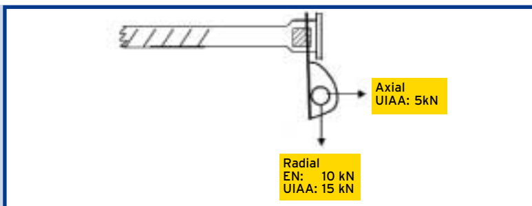
Abb. 1: Vorgeschriebene Bruchwerte laut EN bzw. UIAA- Norm
