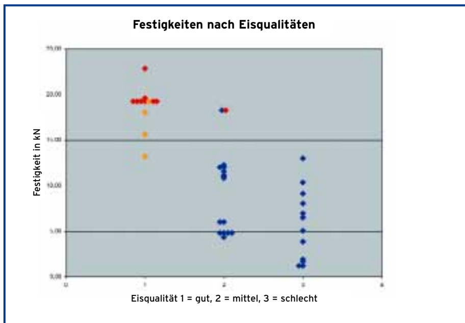
Diagramm 1: Rot: Versuch abgebrochen; gelb: Schraube gebrochen; blau: Eisausbruch.
