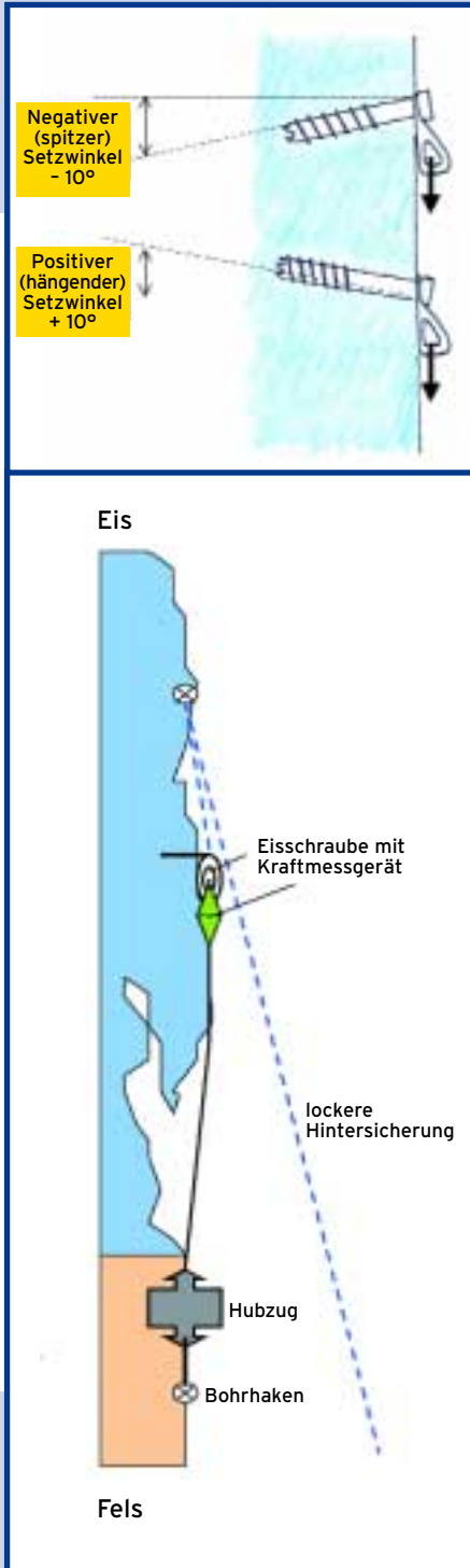
Abb. 3: Der Versuchsaufbau: Mit dem Hubzug ließen sich maximal etwa 20 kN (= 2 Tonnen) erreichen
