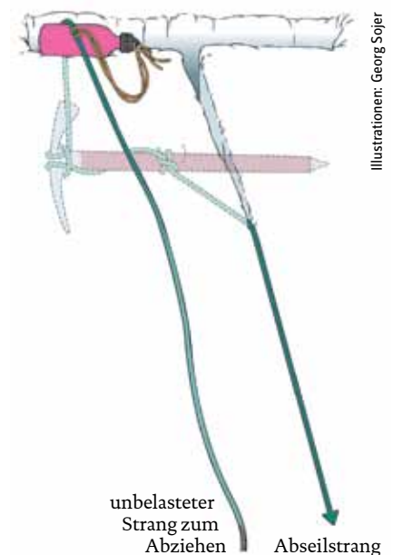
Abb. 3: Der „ausziehbare T-Anker“: clevere Konstruktion zum Abseilen in hartem Firn
