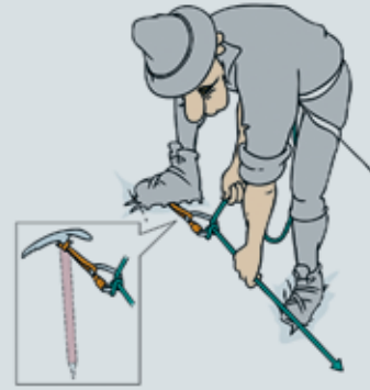
Abb. 2b: „Modifizierter Rammpickel“ im Stehen: die etwas schnellere Variante für Mutige
