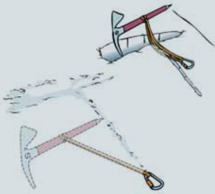
Abb. 1: Der „T-Anker“ mit dem Pickel: etwas aufwändig, aber das Sicherheits-Optimum
